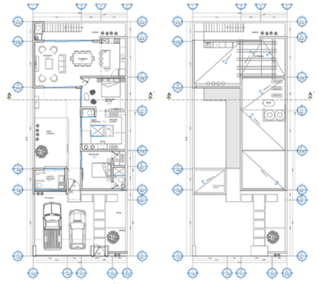
PLANTA ARQUITECTÓNICA 119.61 M 2
